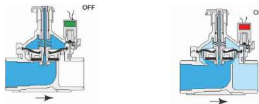
Электромагнитный клапан 2-W
