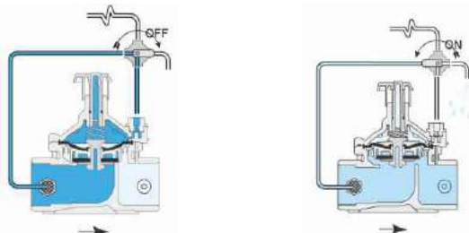
Гидравлический клапан 3-W
