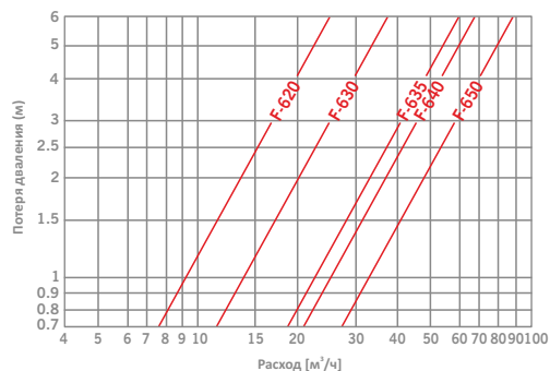
Потеря давления до уровня фильтрации 130 микрон / 120 меш
